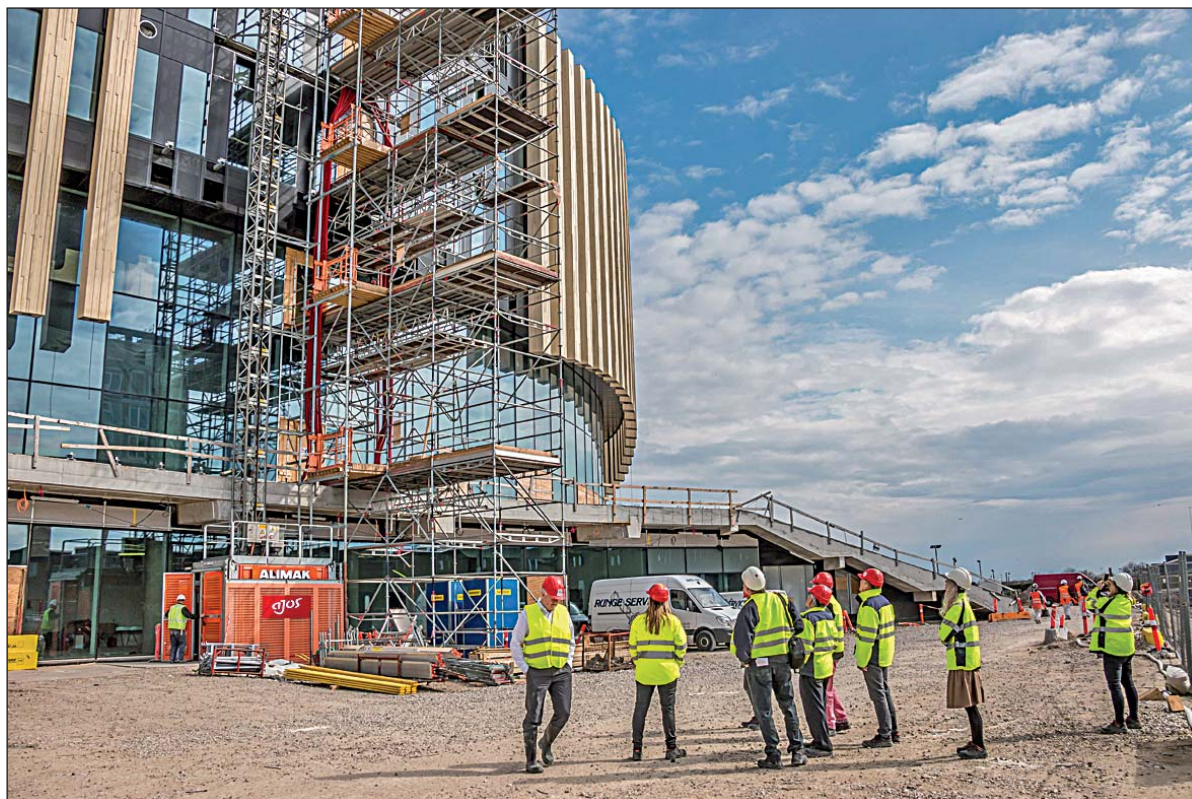
Facaden på Royal Arena tager mere og mere form. Den er beklædt med store lameller af canadisk akoyatræ, som er et meget vejrbestandigt materiale.
